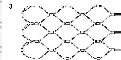
Geschlossene Masche mit Leerhülse, Verbindungsklemme, Sonderrandausbildung Closed mesh with loose ferrule + connection ferrule, special border construction
