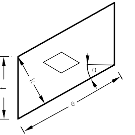
Schrägnetz, Masche horizontal Diagonal mesh panel, horizontal mesh diamond direction
