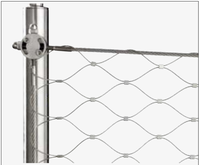
Eckdetail: Anschraubklemme verstellbar Corner detail: adjustable screw-on cross clamp
