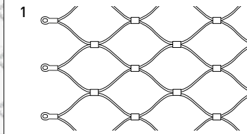
Randausbildung mit Ösen, Standard-Montageart Border construction with eyelets, standard installation
