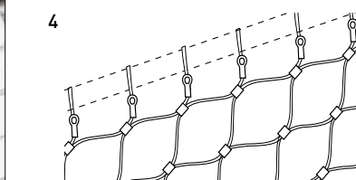
Schräge Randanbindung mit Ösen, Standard Diagonal border construction with eyelets, standard
