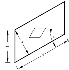
Schrägnetz, Masche parallel zu Ober- / Untergurt liegend Diagonal mesh panel, mesh diamond parallel to top and bottom tubes
