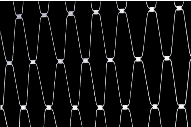
2 Übergroßer Maschenöffnungswinkel, kritische Seilbelastung am Klemmenaustritt, vorrangig für dekorative Anwendungen Oversized mesh opening angle, critical stress on cables at the ferrules' edges, mainly for decorative applications
